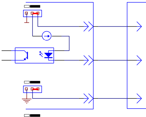
图 6-2 输入信号简化示意图
