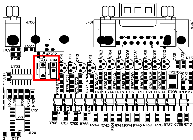
图 6-3 跳线在 Handler 板上的位置
