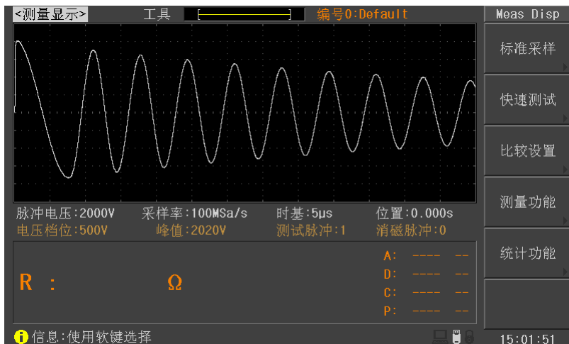
图 4-6-1-1 测量显示页面
