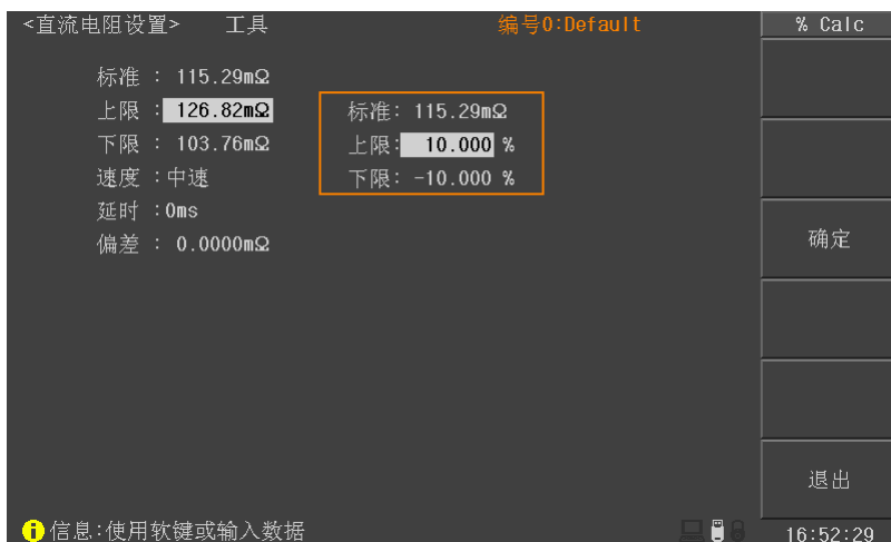
图 4-1-2-4 直流电阻上下限%换算
