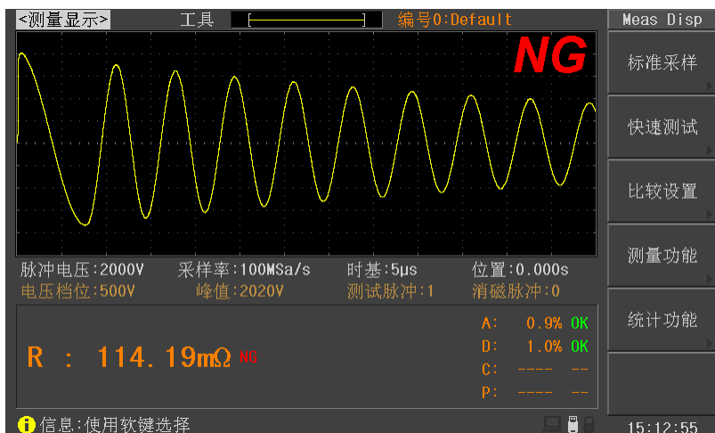
图 4-6-1-2 测量结果显示
